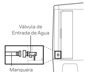
Manguera
